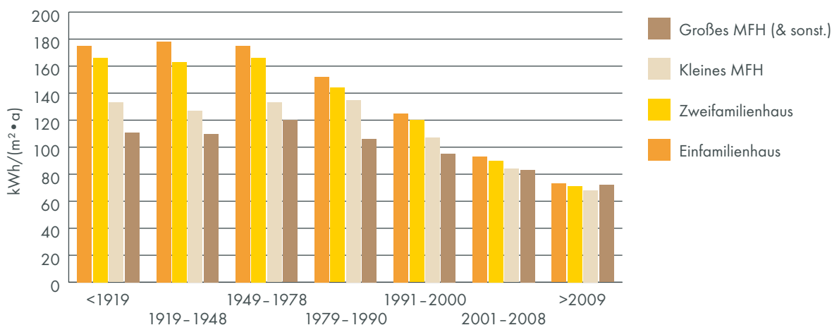
Abbildung 3-31: Wohnimmobilien: Endenergieverbrauchskennwerte für die Beheizung und Warmwasser in kWh/(m 2 •a) bezogen auf die Wohnfläche, nach Gebäudetyp und Altersklassen
