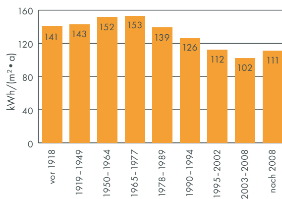
Abbildung 3-32: Büroimmobilien: Endenergieverbrauchskennwerte für die Beheizung und Warmwasser bezogen auf die Nutzfläche, nach Altersklassen
